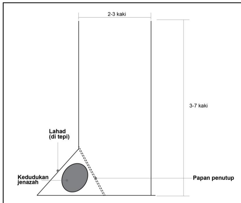
Rajah 2: Jenis Liang Lahad
