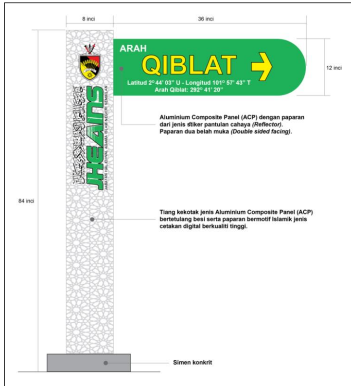
Rajah 1: Ukuran Tanda Arah Kiblat
